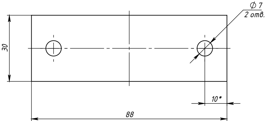
Поз.1 (Полухомут) развертка
